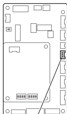
Τερματικό διακόπτη εμπρός (CNA05) Τερματικό αντλίας αποστράγγισης (CN106)
