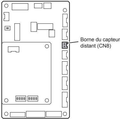
Carte de circuit imprimé de télécommande
